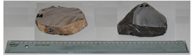
Figure 7. Echantillons pris en surface, 1A : calcaire du Carixien, 2A : calcaire du Bajocien supérieur .
