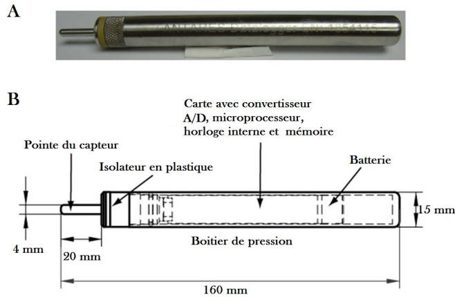
Figure 6. A : Enregistreur de la température (Miniaturized Temperature data Logger (MTL)), B : schéma détaillé d'un MTL (Pfender & Villingner 2002), A/D = analogique-au-digital.
